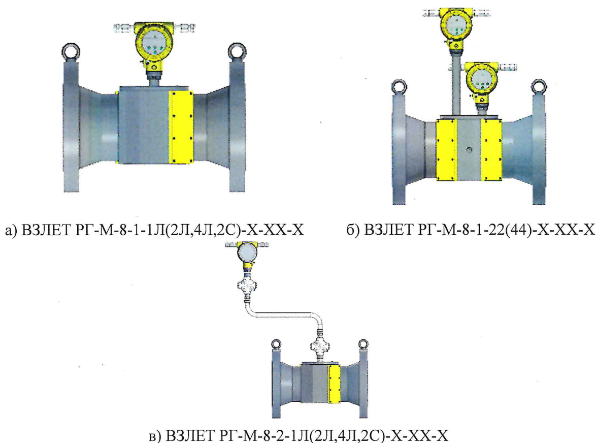
Р и с у н о к 1 – Общий вид расходомеров-счетчиков газа ультразвуковых ВЗЛЕТ РГ-М
