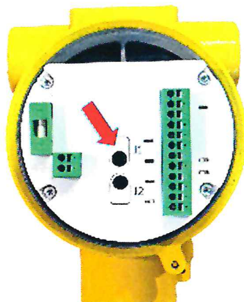
Р и с у н о к 2 – Схема пломбировки от несанкционированного доступа, обозначение места нанесения знака поверки расходомеров-счетчиков газа ультразвуковых ВЗЛЕТ РГ-М
